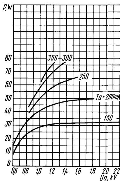
Усредненные характеристики зависимости колебательной мощности от напряжения анода в режиме непрерывного генерирования: \lambda = 18.5 см Averaged Characteristic Curves Showing Oscillator Output Power versus Anode Voltage in Continuous-Wave Generation: \lambda = 18.5 cm
