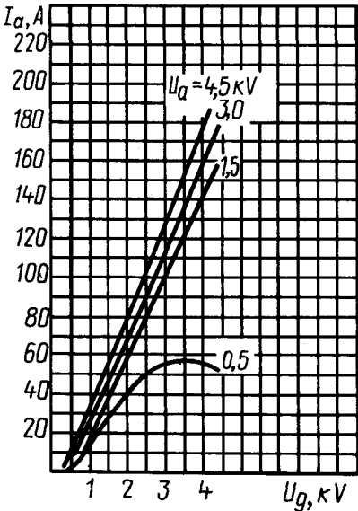
Усредненные анодно-сеточные характеристики: U_i = 6.3\text{ В} Averaged Anode-Grid Characteristic Curves: U_i = 6.3\text{ В}
