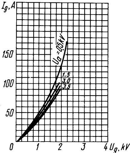
Усредненные сеточные характеристики: U_i = 6.3\text{ В} Averaged Grid Characteristic Curves: U_i = 6.3\text{ В}
