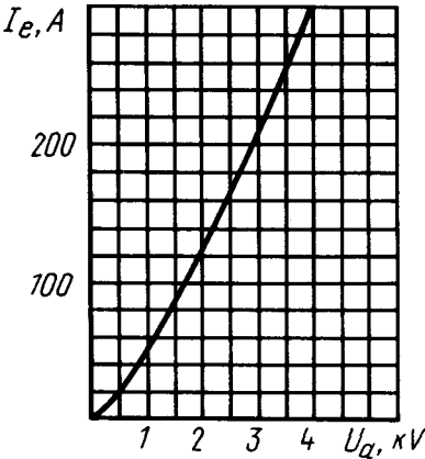
Усредненная эмиссионная характеристика: U_i = 6.3\text{ В} Averaged Emission Characteristic Curves: U_i = 6.3\text{ В}
