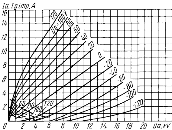
Усредненные импульсные характеристики: U_i = 12,6 \text{ В} ; \tau = 2 \text{ мкс} ; частота посылок ( f_i ) равна 1000 имп/с; ————— анодные; - - - - - сеточно-анодные Averaged Peak Characteristic Curves: U_i = 12.6 \text{ V} ; \tau = 2 \mu\text{s} frequency 1,000 imp/s: ————— anode; - - - - - grid-anode
