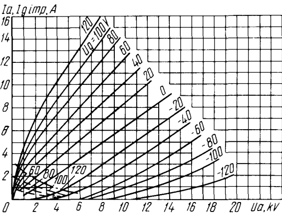
Усредненные импульсные характеристики: U_i = 12,6 \text{ В} ; \tau = 2 \text{ мкс} ; частота посылок ( f_i ) равна 1000 имп/с; ——— анодные; ----- сеточно-анодные Averaged Peak Characteristic Curves: U_i = 12.6 \text{ V} ; \tau = 2 \mu\text{s} frequency 1,000 imp/s: ——— anode; ----- grid-anode
