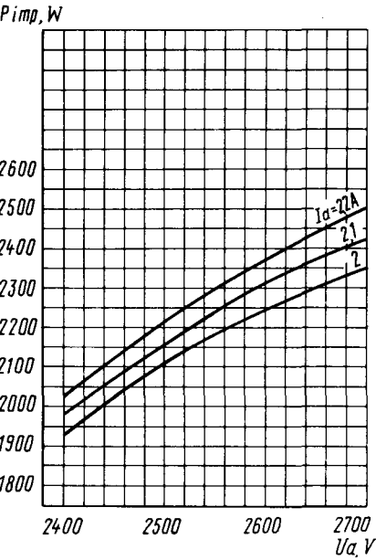
Усредненные характеристики зависимости колебательной мощности в импульсе от напряжения анода: U_g = 6,3\text{ В} Averaged Characteristic Curves Showing Peak Oscillator Output Power versus Anode Voltage: U_g = 6.3\text{ V}
