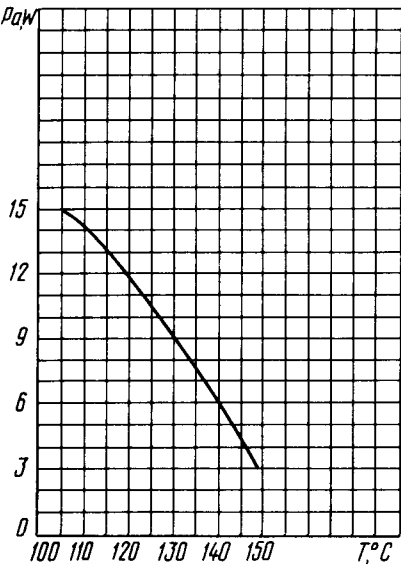
Зависимость мощности, рассеиваемой анодом, от температуры окружающей среды температур баллона (T б ) при равной 200 °C Characteristic Curves Showing Anode Dissipation P a max versus Ambient Temperature (at bulb temperature T b 200 °C)
