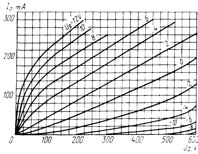
Усредненные анодные характеристики Averaged Anode Characteristic Curves
