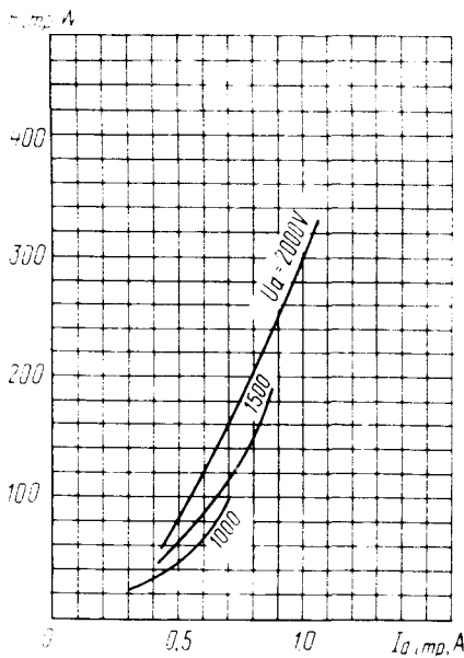
Характеристики зависимости выходной мощности от тока анода в импульсе: U_i = 12,6 \text{ В} ; \tau = 2 \text{ мкс} ; частота посылок ( f_r ) равна 500 Гц Characteristic Curves Showing Output Power versus Peak Anode Current: U_i = 12,6 \text{ В} ; \tau = 2 \text{ мкс} pulse frequency 500 Hz
