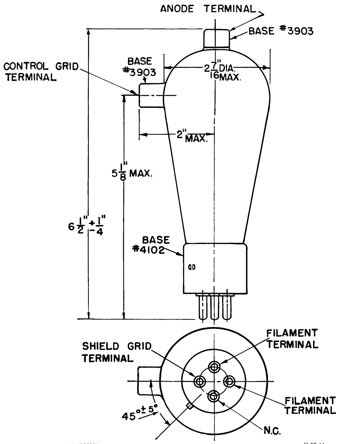
OUTLINE FG-98-A THYRATRON
