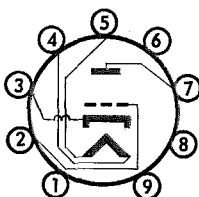
Pentode F 7024 L
