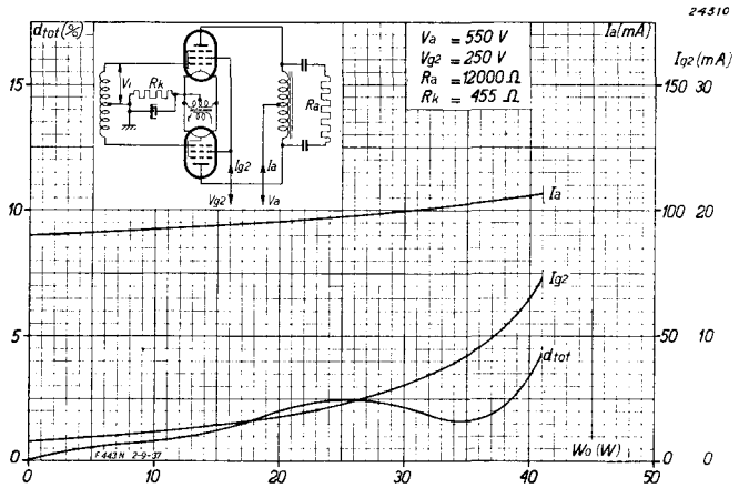
Abb. 11 Gesamtverzerrung, Gesamtanodenstrom und Gesamtschirmgitterstrom als Funktion der Ausgangsleistung bei Verwendung von zwei Röhren F 443 N in Gegentakt mit automatischer Gittervorspannung und bei V_a = 550 V, V_{g2} = 250 V.
