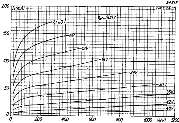
Abb. 6 Anodenstrom als Funktion der Anodenspannung bei V_{g2} = 200 V mit der negativen Gitterspannung als Parameter.
