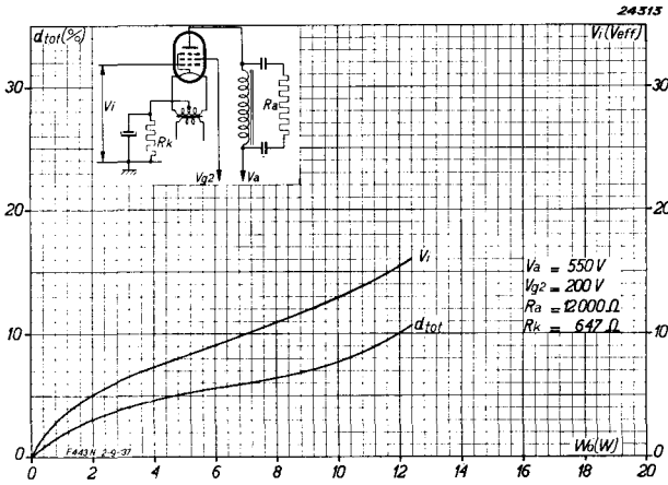
Abb. 8 Gesamtverzerrung und Gitterwechselspannungsbedarf als Funktion der Ausgangsleistung bei V_a = 550 V und V_{g3} = 200 V und bei Verwendung der Röhre F 443 N als einfache Endröhre.
