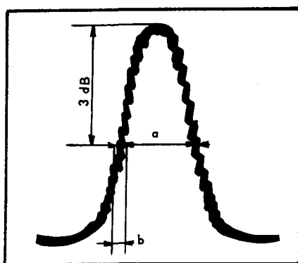
Fig. 4 f_m \simeq 5 kHz, \Delta f = 1,400 \times \frac{b}{a} \simeq 0,15 MHz défaut caractérisé.
