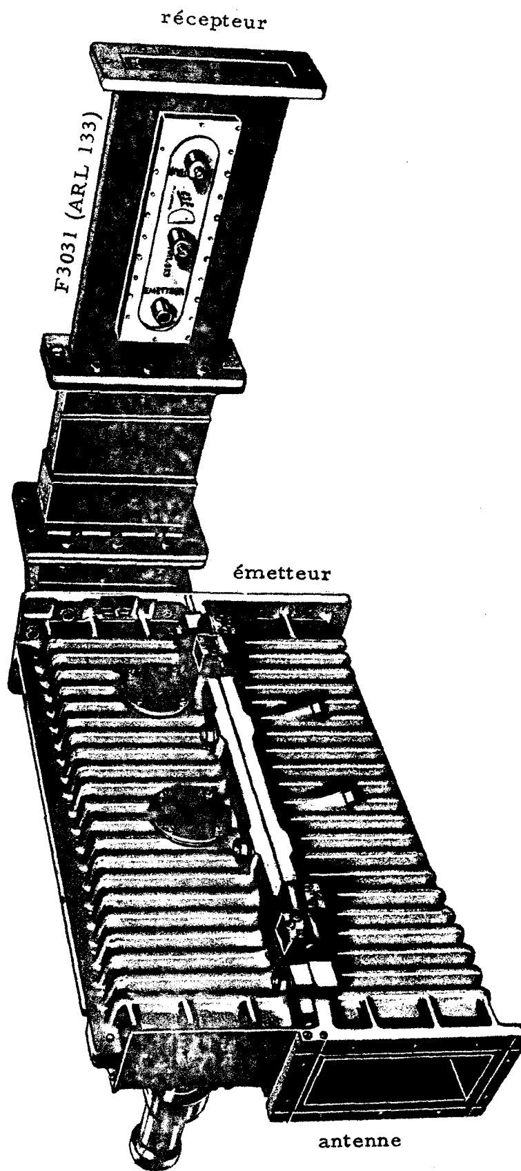
DUPLIXEUR F 3023 (AP 623) AVEC TUBE F 3031 (ARL 133)
