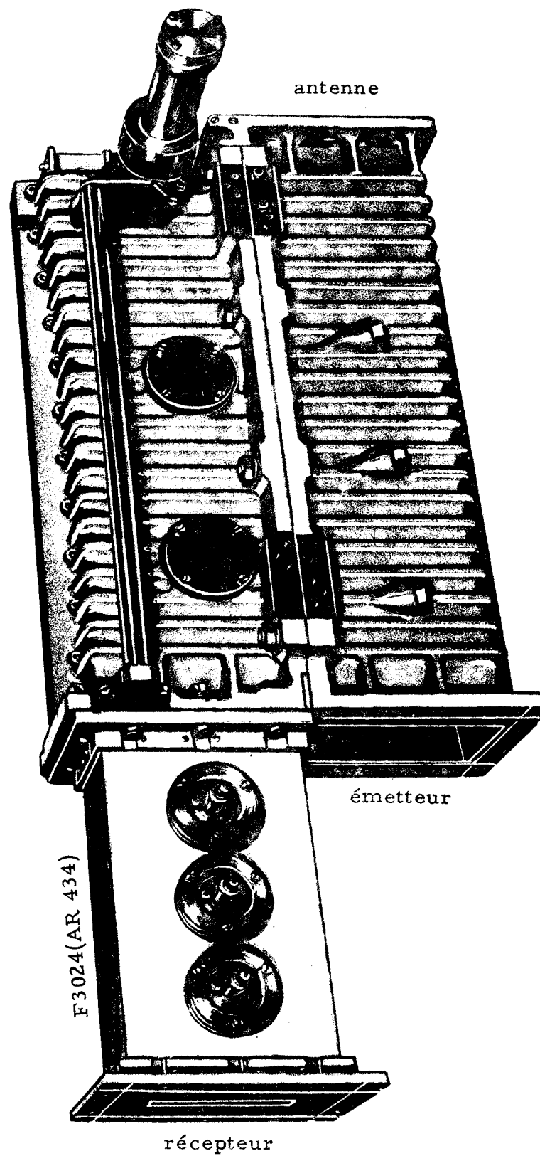
DUPLExEUR F 3023(AP 623) AVEC MONTURE F 3024(AR 434)
