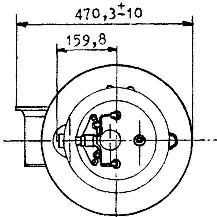
TUBE NU
