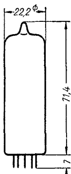
max. Abmessungen
