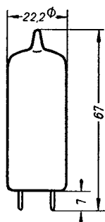
Kolbenabmessungen
