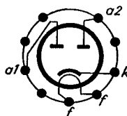
Sockelschaltschema
