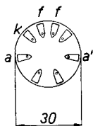
Abb. 2 Elektrodenanordnung und Sockelanschlüsse.
