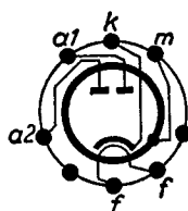
Sockelschaltschema
