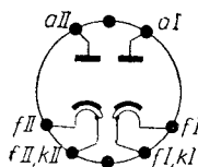
Sockelschaltchema
