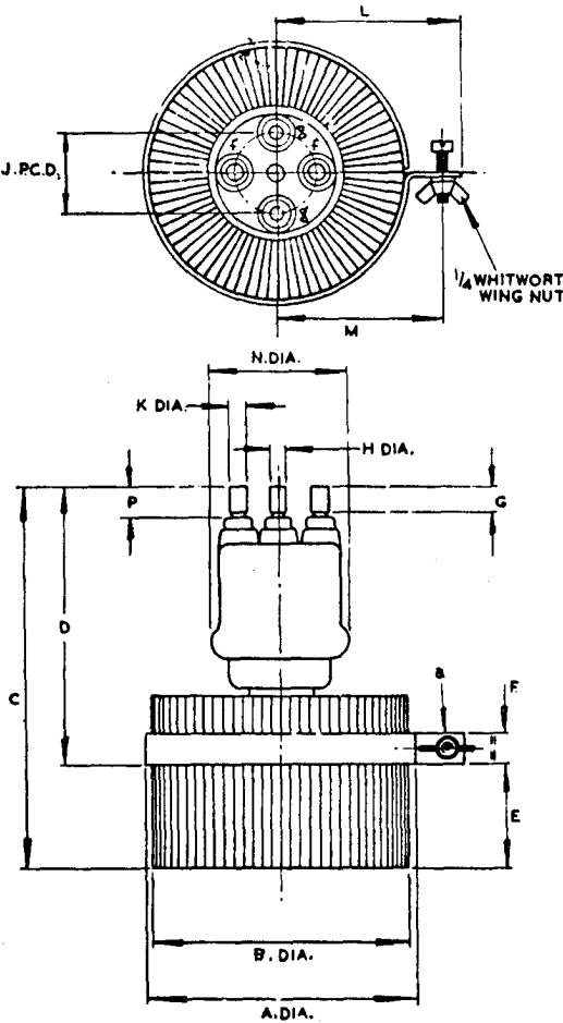
ESA1500 Outline
