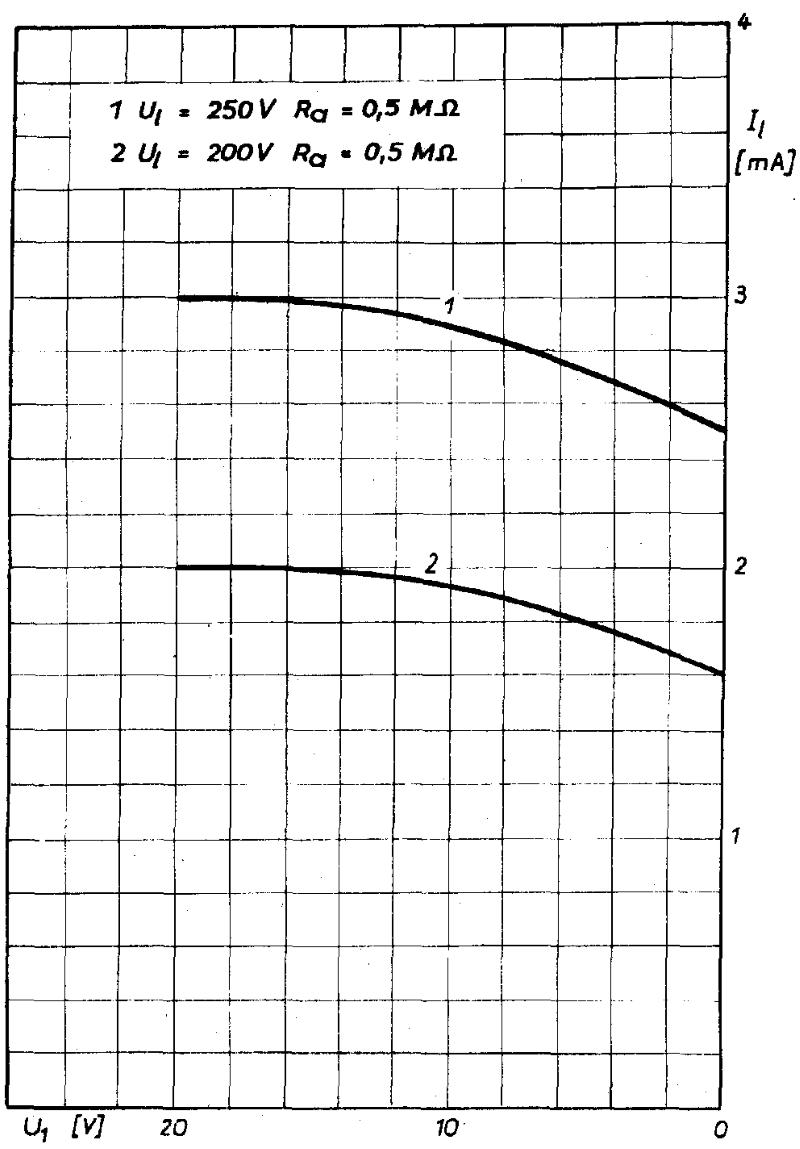
Leuchtschirmstrom als Funktion der Gitterspannung
