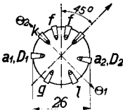
Abb. 2 Elektrodenanordnung und Sockelanschlüsse. l = Fluoreszenzschirm.
