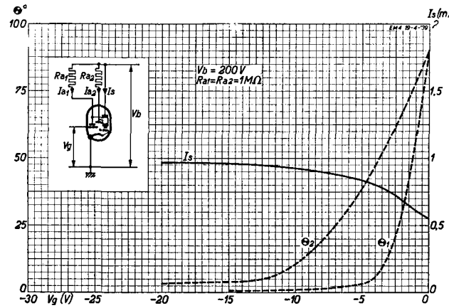
Abb. 7 Schattenwinkel \Theta_1 und \Theta_2 , gemessen am Rande des Schirmes, und Schirmstrom I_s als Funktion der Gitterspannung bei einer Speisespannung von 200 V.
