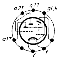
Sockelschaltchema
