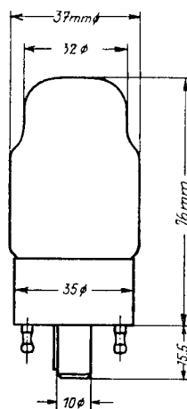
Kolbenabmessungen
