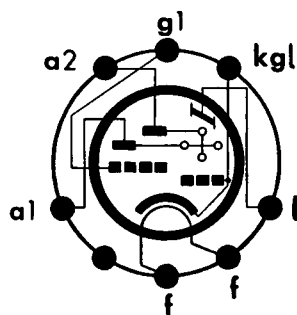
Sockelschaltbild
