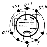
Sockelschaltschema
