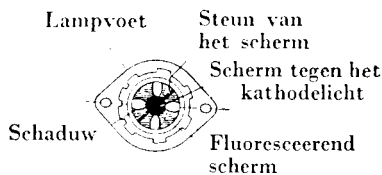
Vooraanzicht van het afstemkruis.
