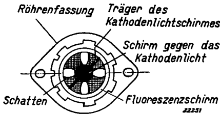
Abb. 5 Kopfansicht des Abstimmkreuzes mit Röhrenfassung. Die Trägerstange des Kathodenlichtschirmes gibt die Richtung des Kreuzes an.
