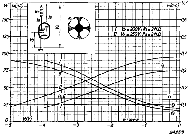
Abb. 3 Anodenstrom des Triodenteiles I_a , Strom zum Fluoreszenzschirm I_s und Lichtwinkel \Theta , gemessen am Rande des Schirmes als Funktion der negativen Gitterspannung bei V_b = 200\text{ V} (Kurve I) und V_b = 250\text{ V} (Kurve II).
