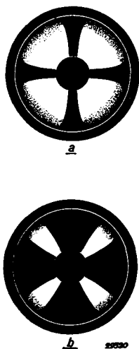
Abb. 4 a) Lichtbedeckung des Fluoreszenzschirmes bei großer negativer Spannung am Gitter des Triodenteiles. b) Lichtbedeckung des Fluoreszenzschirmes bei kleiner negativer Spannung am Gitter des Triodenteiles.
