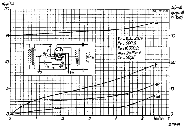
Abb. 5 Gesamtverzerrung d_{tot} , Gitterwechselspannungsbedarf pro Gitter V_i , Gesamtanodenstrom I_a und Gesamtschirmgitterstrom I_{g2} als Funktion der Ausgangsleistung bei Verwendung der ELL 1 als Gegentaktverstärker mit automatischer Vorspannung.
