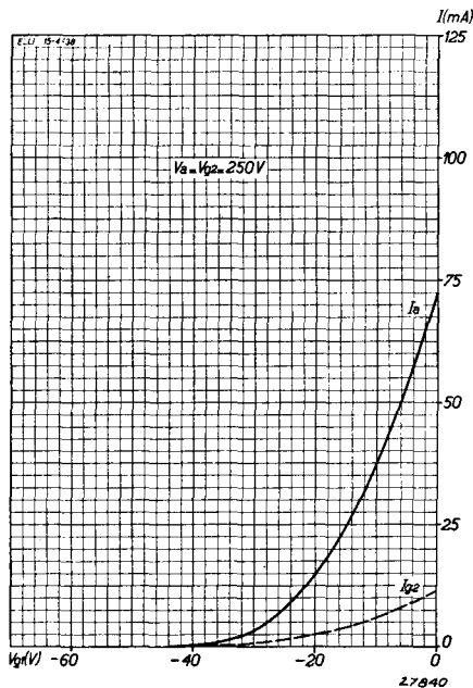
Abb. 3 Anodenstrom und Schirmgitterstrom eines Penthodensteiles der ELL 1 als Funktion der negativen Gitterspannung bei V_a = V_{g2} = 250 \text{ V} .
