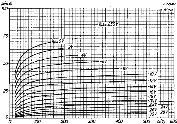
Abb. 4 Anodenstrom eines Penthodenröhre als Funktion der Anoden- spannung bei verschiedenen negativen Gitterspannungen und V_{g2} = 250 V.
