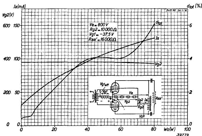
Fig. 12 Dezelfde krommen als in fig. 9, echter voor het geval, dat de schermroosterspanning via een serie weerstand van 8 000 \Omega van de voedingspanning van 800 V wordt afgenomen en met behulp van vier stabiliseerbuisen 13201 constant wordt gehouden.
