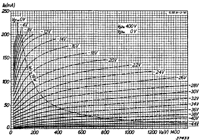
Fig. 5 Anodestroom als functie van de anodespanning bij V_{g2} = 400 V en met V_{g1} als parameter (800 V instelling).
