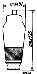
Fig. 1 Afmetingen in mm.
