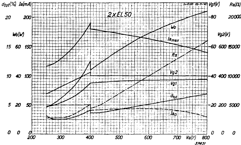
Fig. 11 Maximum anodestroom I_{a_{max}} , anoderuststroom I_{a_0} , schermroosterspanning V_{g_2} , negatieve roosterspanning V_{g_1} , geleverd vermogen W_o , totale vervorming d_{tot} en gunstigste belastingsimpedantie R_a , als functie van de beschikbare anodespanning V_a voor twee in balans geschakelde buizen EL 50 met vaste negatieve roosterspanning.
