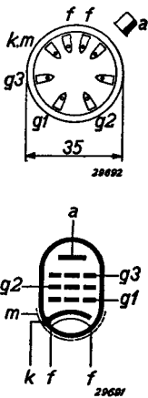
Fig. 2 Rangschikking van de electroden en aansluitingen van de huls.
