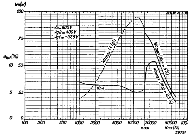
Fig. 10 Maximum geleverd vermogen W_o als functie van de belastingimpedantie R_{aa'} voor twee in balans geschakelde buizen EL 50 met vaste negatieve roosterspanning en bij V_a = 800 V, V_{g_1} = 400 V, en V_{g_1} = -37,5 V. De gestippelde lijn W_o \max (+I_{g_1}) stelt de grens voor, waarbij de buis juist tot het optreden van roosterstroom wordt gemoduleerd. In dit geval zou de maximum anodedissipatie echter worden overschreden.
