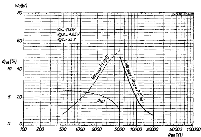
Fig. 8 Maximum geleverd vermogen W_o als functie van de belastingimpedantie R_{aa'} voor twee in balans geschakelde buizen EL 50 met vaste negatieve rooster spanning en bij V_a = 400V , V_{g2} = 425V en V_{g1} = -35V . De gestippelde lijn W_{omax} (+I_{g2}) stelt de grens voor, waarbij de buis juist tot het optreden van roosterstroom wordt gemoduleerd. In dit geval zou de maximum anodedissipatie echter worden overschreden.
