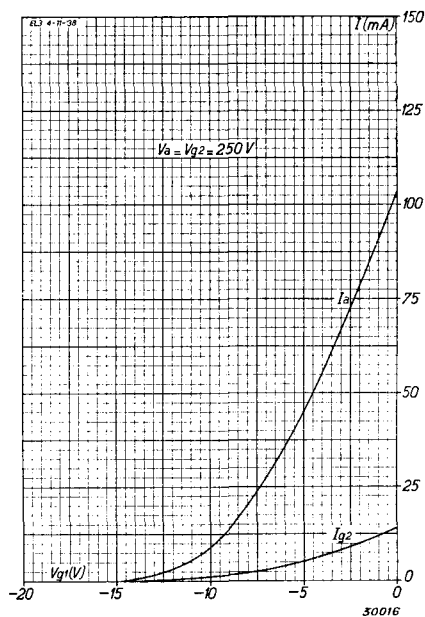
Abb. 4 Anodenstrom als Funktion der negativen Gitterspannung bei V_a = V_{g2} = 250 \text{ V} .
