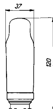
Encombrement du tube EL 3. Fig. 6
