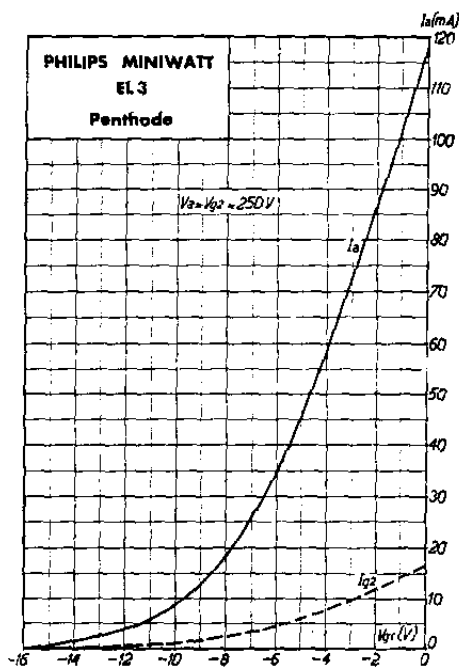
Courant anodique et courant de grille-écran en fonction de la polarisation négative de la grille pour V_a = V_{g2} = 250 volts.
