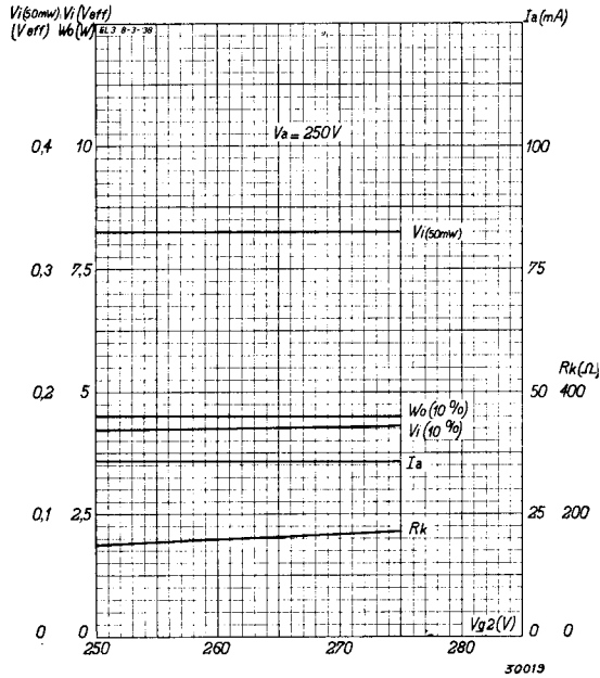
Abb. 7 Ausgangsleistung bei 10 % Verzerrung . . . W_o (10 %) Gitterwechselspannungsbedarf bei 10 % Verzerrung . . . V_i (10 %) Empfindlichkeit . . . . . V_i (50 mW) Kathodenwiderstand . . . . . R_k Anodenstrom . . . . . I_a als Funktion der Schirmgitterspannung (in einem Bereiche von 250 bis 275 V) bei konstanter Anodenspannung ( V_a = 250 V).
