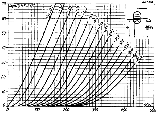
Abb. 6 Anodenstrom als Funktion der Anodenspannung bei verschiedenen negativen Gitterspannungen, wenn die EL 2 als Triode verwendet wird.
