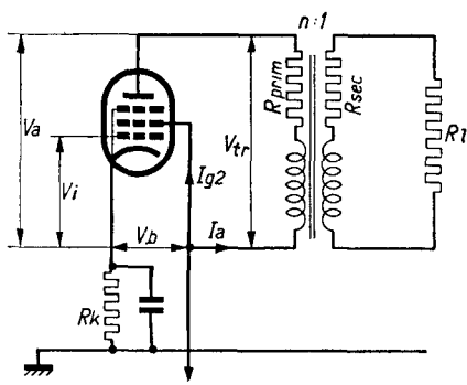
Abb. 11 Schaltung der Röhre EL 2, mit der die Messungen der Tabelle II durchgeführt wurden. Wegen der verschiedenen Bezeichnungen und Formeln siehe die Unterschrift der Abb. 10.
