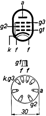
Abb. 2 Elektrodenanordnung und Sockelanschlüsse.
