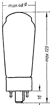
Kolbenabmessungen
