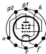
Sockelschaltchema
