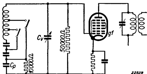
Abb. 13 Schaltung des Oszillatorkreises bei Verwendung eines kleineren Ableitwiderstandes unter Berücksichtigung des kleinen Wertes des Paddingkondensators auf Lang- und Mittelwellen.
