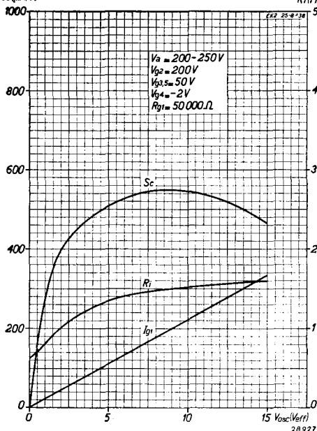
Abb. 4 Mischsteilheit S_c , Innenwiderstand R_i und Oszillatorgitterstrom I_{g1} als Funktion der Oszillatorspannung bei V_{g2} = 200 V und V_{g3,5} = 50 V.
