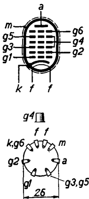
Abb. 2 Elektrodenanordnung und Sockelanschlüsse.
