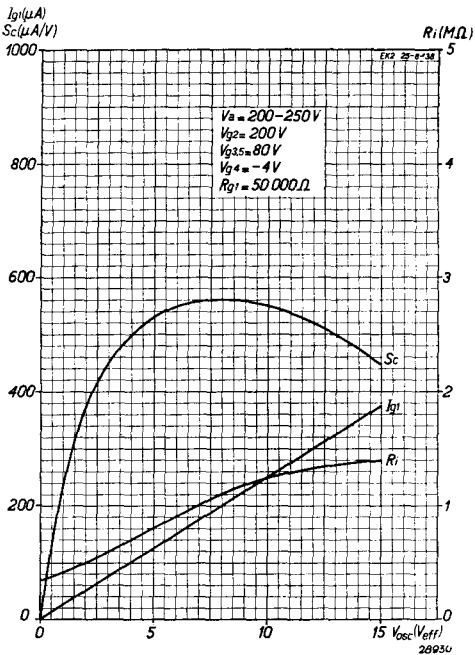
Abb. 5 Mischsteilheit S_c , Innenwiderstand R_i und Oszillatorgitterstrom I_{g1} als Funktion der Oszillatorspannung bei V_{g2} = 200 V und V_{g3,5} = 80 V.
