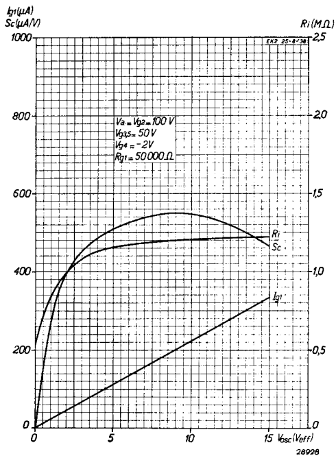
Abb. 7 Mischsteilheit S_c , Innenwiderstand R_i und Oszillatorgitterstrom I_{g1} als Funktion der Oszillatorspannung bei V_{g_3} = 100V und V_{g_{3,5}} = 50V .
