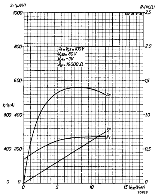
Abb. 6 Mischsteilheit S_c , Innenwiderstand R_i und Oszillatorgitterstrom I_{g1} als Funktion der Oszillatorspannung bei V_{g_3} = 100V und V_{g_{3,5}} = 80V .
