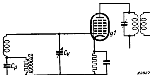
Abb. 12 Schaltung bei Verwendung eines kleineren Ableitwiderstandes, wenn sich der Paddingkondensator in Serie mit der Spule befindet.
