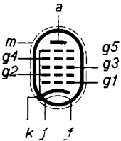
Abb. 2 Elektrodenanordnung und Sockelanschlüsse.
