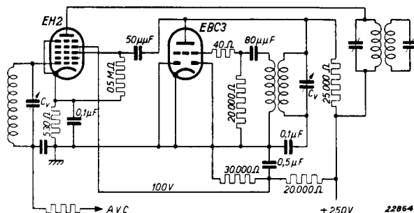
Abb. 10 Prinzipialschaltung für die Verwendung der Röhre EH 2 als Mischröhre mit der EBC 3 als Oszillator.
