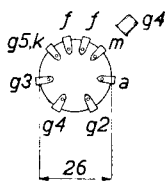
Abb. 1 Abmessungen in mm.
