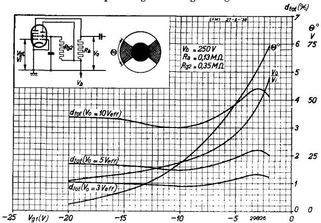
Abb. 5 Verzerrung als Funktion der Gittervorspannung mit der Ausgangswechselspannung als Parameter bei R_{g2} = 350.000 Ohm, R_a = 130.000 Ohm und V_b = 250 V und Schattenwinkel \Theta als Funktion der Gittervorspannung.
