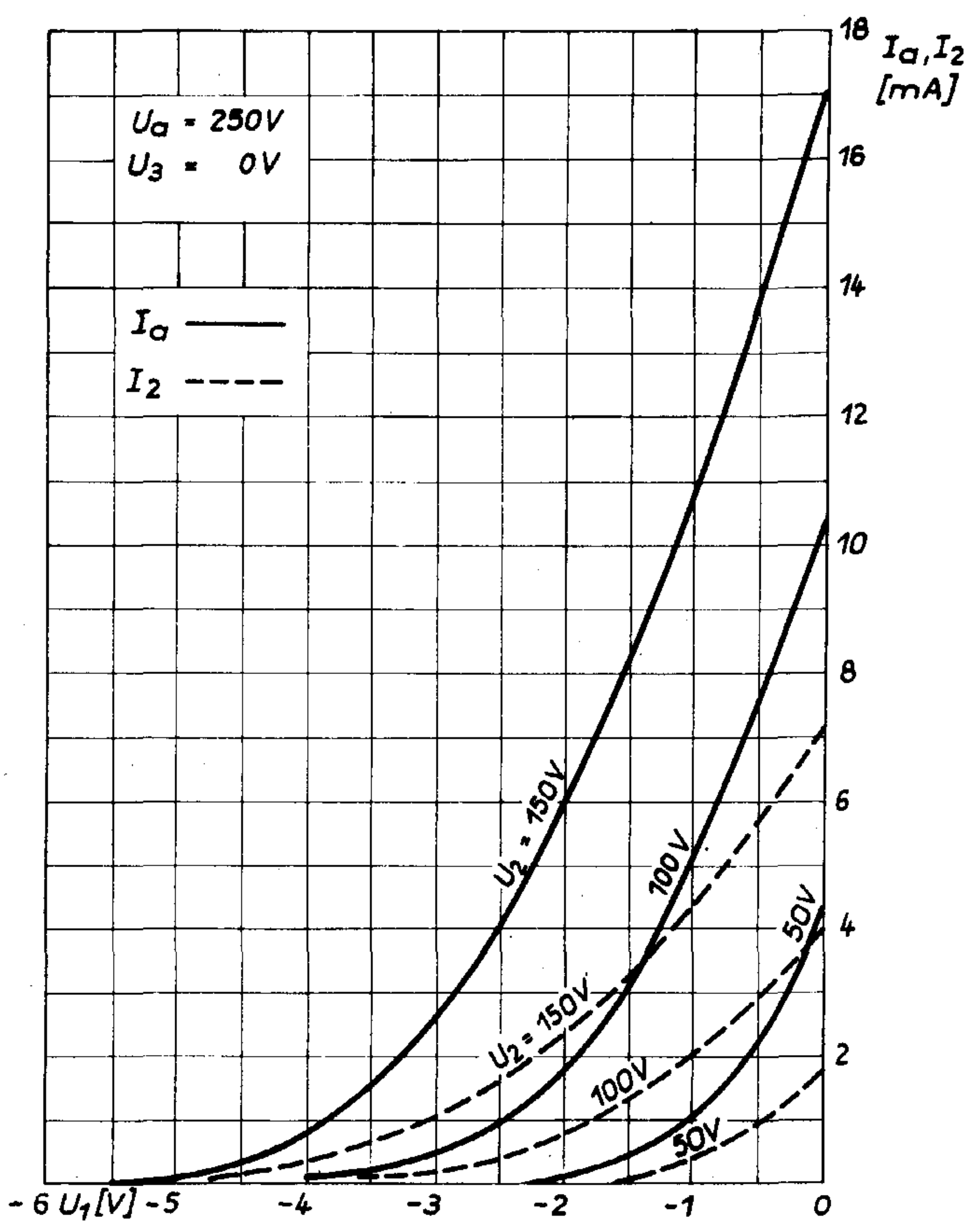
Anodenstrom und Schirmgitterstrom als Funktion der Gittervorspannung
