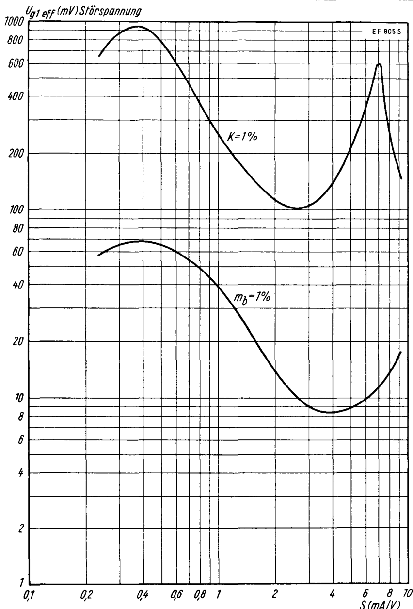
Kurven für Kreuz- und Brumm-Modulation Characteristic curves for cross and hum modulation Courbes pour transmodulation et modulation par ronflement U_b=200\text{ V} , R_{g2}=45\Omega , U_{g3}=0\text{ V}
