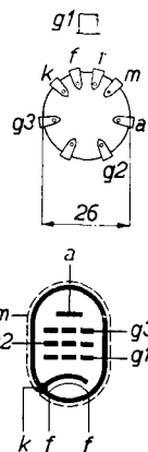
Abb. 2 Elektrodenanordnung und Sockelanschlüsse.
