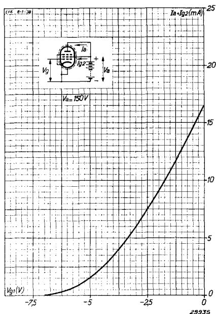
Abb. 5 Anodenstrom als Funktion der negativen Gitterspannung bei Verwendung der EF 6 als Triode.
