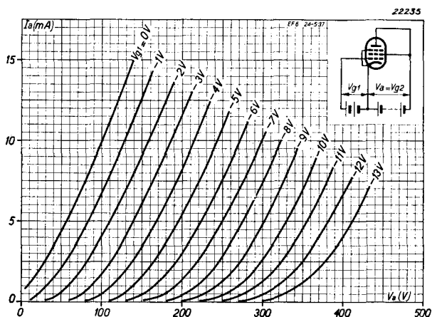
Abb. 6 Anodenstrom als Funktion der Anodenspannung bei verschiedenen negativen Gitterspannungen bei Verwendung der EF 6 als Triode.
