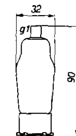
Encombrement du tube EF6.
