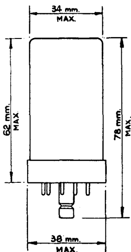
DIMENSIONS
