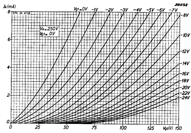
Abb. 9 Anodenstrom als Funktion der Schirmgitterspannung für verschiedene negative Gitterspannungen.
