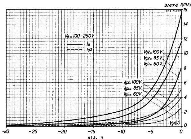
Abb. 3 Anodenstrom und Schirmgitterstrom als Funktion der Steuergitterspannung für drei verschiedene Schirmgitterspannungen und für eine Anodenspannung von 250 Volt. Die Kurven gelten annähernd für alle Anodenspannungen zwischen 100 und 250 Volt.
