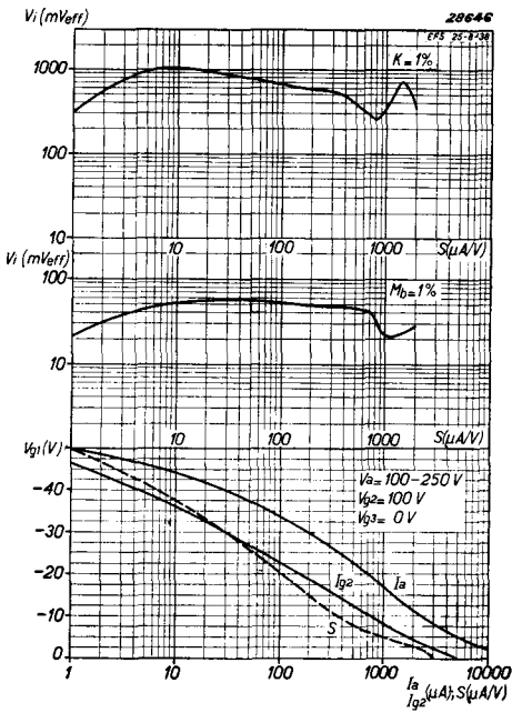
Abb. 5 Für eine Schirmgitterspannung von 100 V : Obere Kurve: Effektive Gitterwechselspannung als Funktion der Steilheit für 1% Quermodulation. Mittlere Kurve: Effektive Gitterwechselspannung als Funktion der Steilheit für 1% Modulationsbrummen. Untere Kurven: Steilheit S und Ia als Funktion der Spannung des ersten Gitters.
