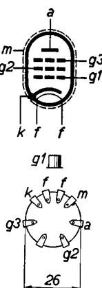
Abb. 2 Elektrodenanordnung und Sockelanschlüsse.
