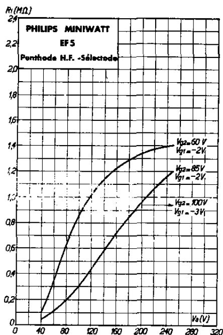
Résistance interne en fonction de la tension d'anode pour 3 tensions différentes de grille-écran avec les polarisations de la grille 1 correspondantes. Les courbes de V_{g2} = 85 \text{ V} , V_{g1} = -2 \text{ V} et V_{g2} = 100 \text{ V} , V_{g1} = -3 \text{ V} coïncident en pratique complètement.
