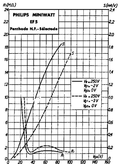
Résistance interne et pente en fonction de la tension de grille-écran pour une tension d'anode fixe et deux polarisations différentes de la grille 1.
