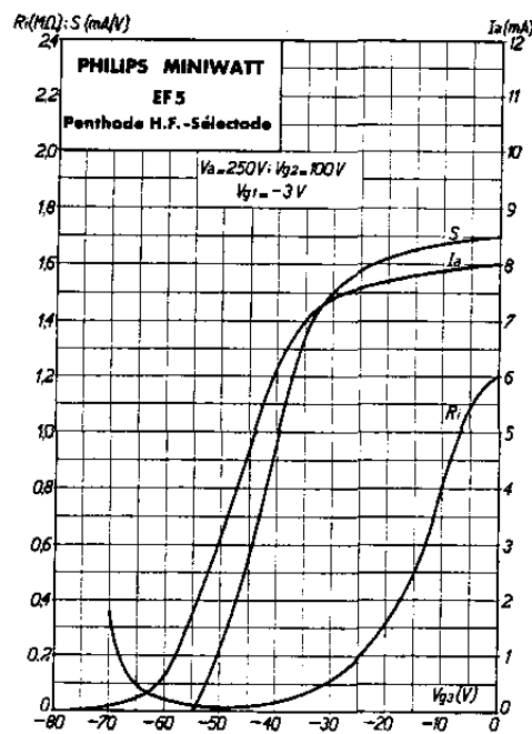
Résistance interne R_i , pente S et courant d'anode I_a en fonction de la tension négative sur la grille 3 pour V_a = 250 \text{ V} , V_{g2} = 100 \text{ V} et V_{g1} = -3 \text{ V} .
