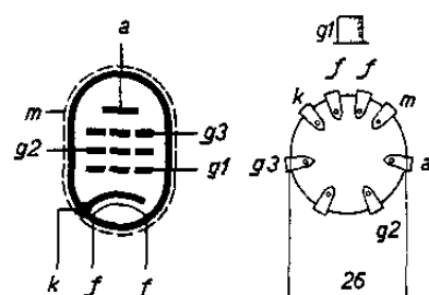
Disposition des électrodes et connexions du culot.
