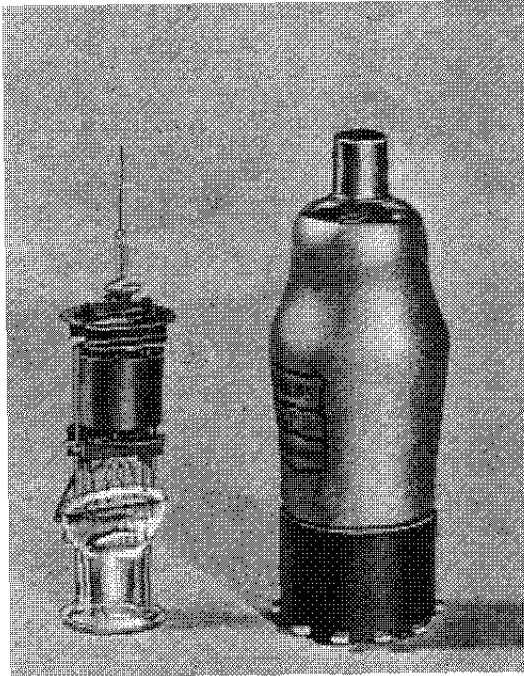
La nouvelle penthode-sélectode EF 5 et sa construction interne.
