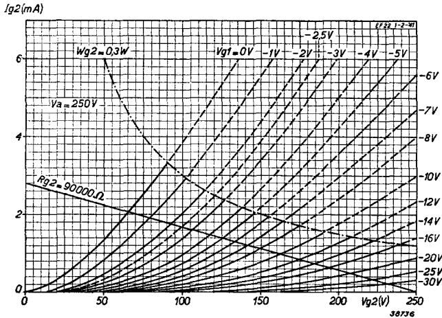
Fig. 8 Schermroosterstroom als functie van de schermroosterspanning bij V_a = 250 \text{ V} met de negatieve roosterspanning als parameter. In de kromme is tevens de belastinglijn voor den schermrooster-serieweerstand R_{g2} = 90\,000 \Omega geteekend.
