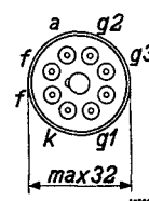
Fig. 2 Rangschikking en aansluitingen van de elektroden.
