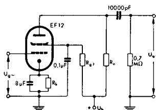
Schaltung für NF-Verstärker mit Widerstandskopplung
