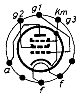
Sockelschaltchema
