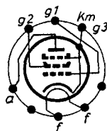
Sockelschaltchema
